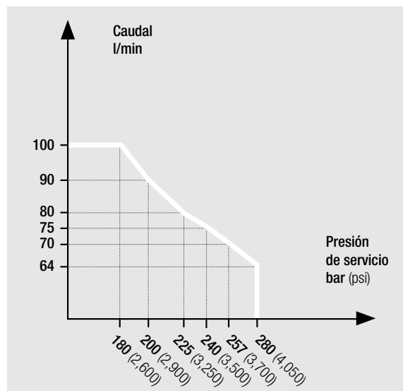
CAUDAL - PRESIÓN DE SERVICIO, 1 ER . CIRCUITO PARA DISPOSITIVOS AUXILIARES (PROPORCIONAL)
